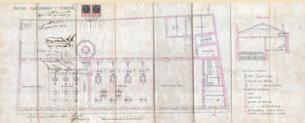
Plán elektrárny z 21. 3. 1892. Podepsán starostou města F. Bláhou. Na technickém výkresu jsou ve strojovně narysovány 4 parní kotle, 4 dynamy pro žárovky a 4 dynamy určená pro obloukové lampy. (reprofoto z knihy: Antl – Vík, Křižkova žižkovská elektrárna. Praha 2024)
